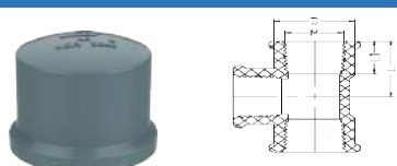
End Cap
