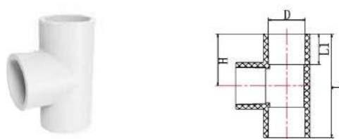
Tee
